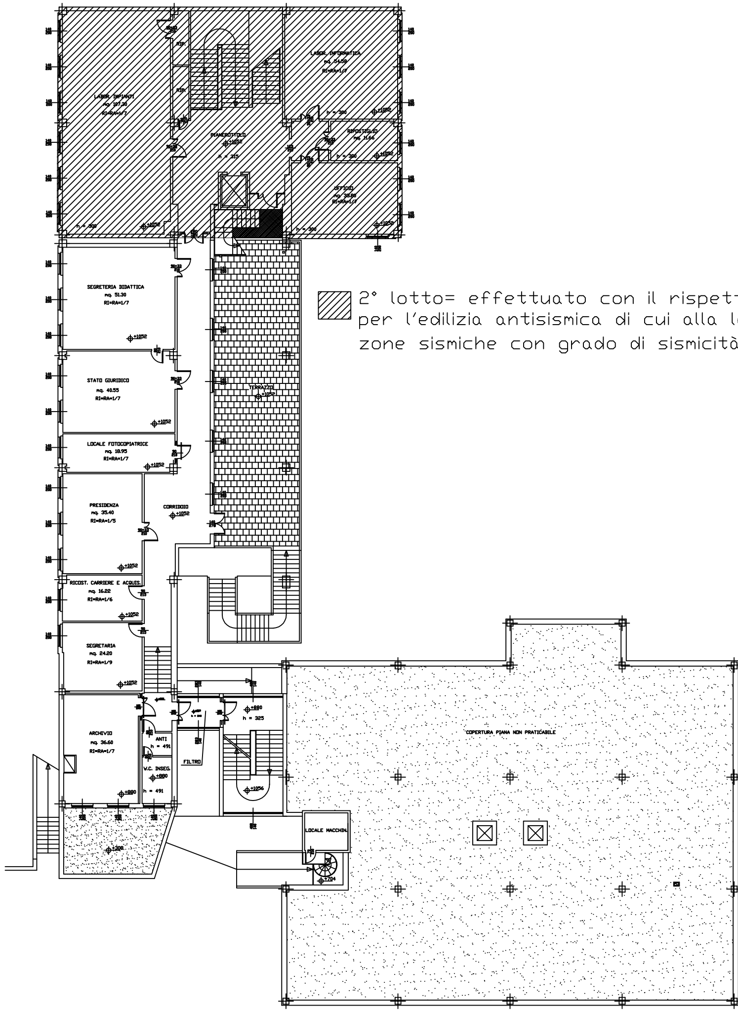
PIANO TERZO
